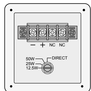
Beispiel: eingestellte Nennbelastung = 12,5W Example: rated load adjusted = 12.5W
